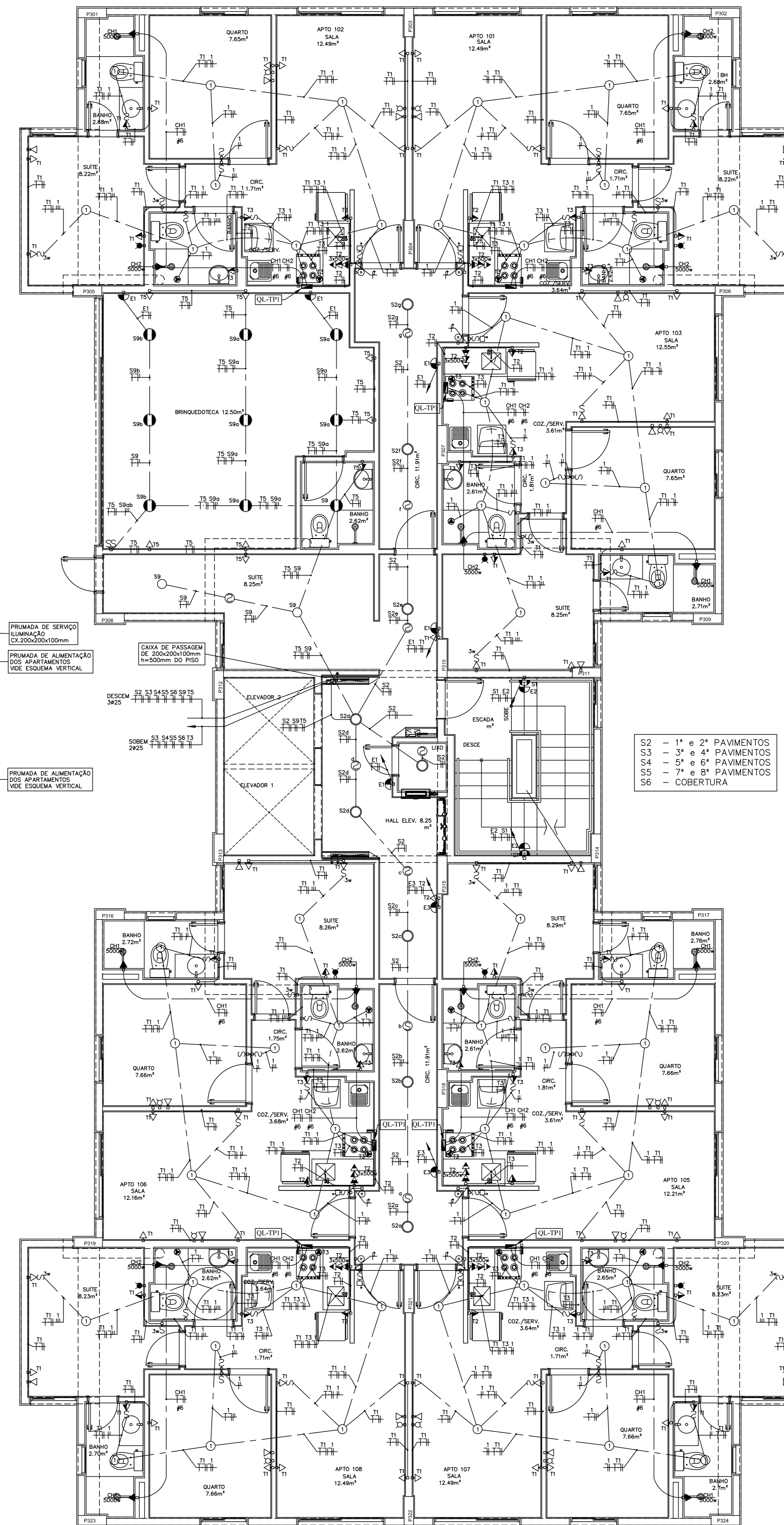
PLANTA BAIXA 1º PAVIMENTO BLOCO C ESCALA 1:50
