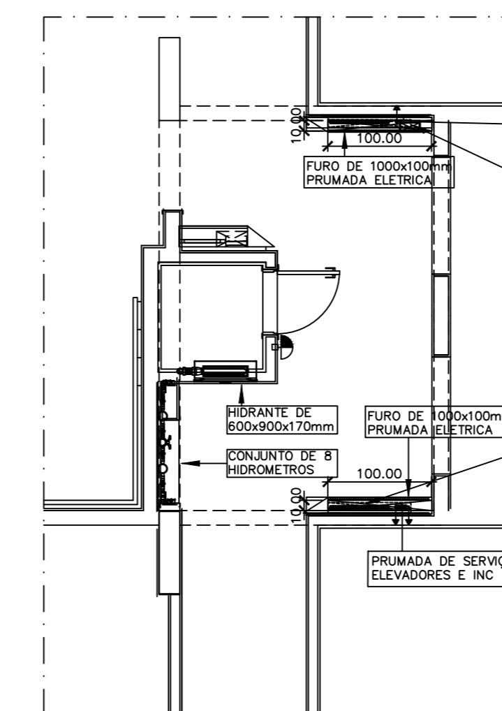
PRUMADAS NO PAVTO.TIPO ESCALA 1:50
