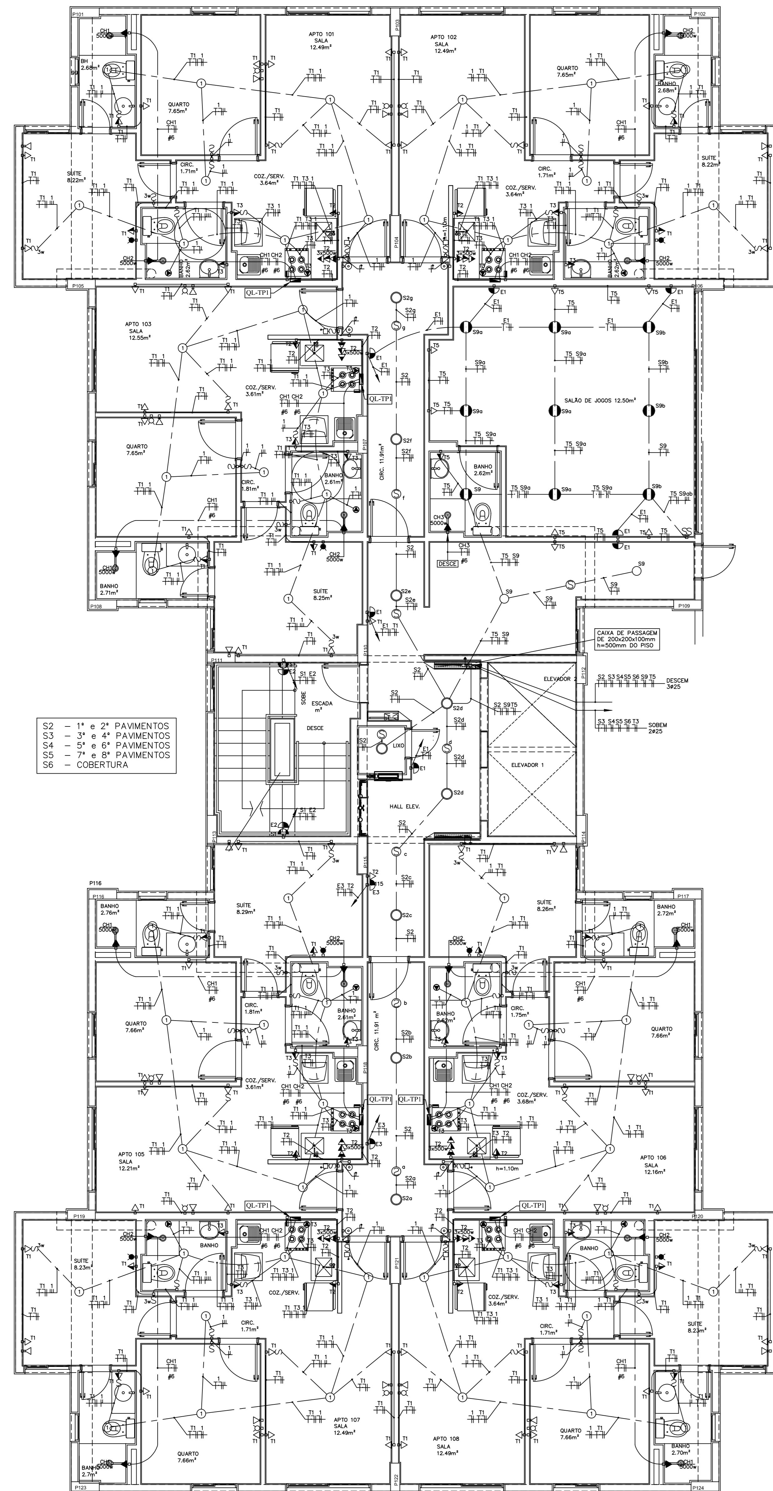
PLANTA BAIXA 1º PAVIMENTO BLOCO A ESCALA 1:50
